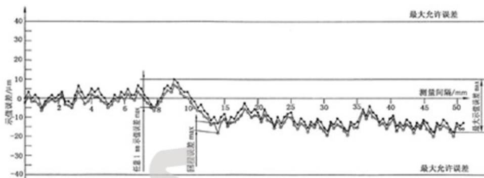
图5 量程超过10 mm的指示表,已设定零位的示值误差曲线示意图
